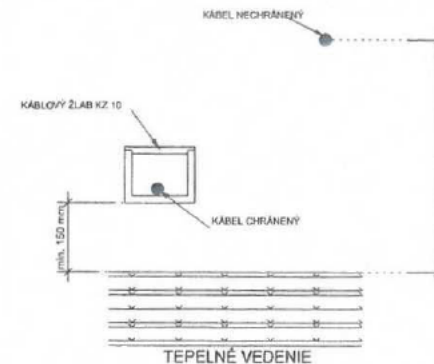
NAJMENŠIE DOVOLENÉ VZDIALENOSTI PRI SÚBEHU A KRIŽOVANÍ PODZEMNÝCH VEDENÍ v m PODĽA STN 73 6005
