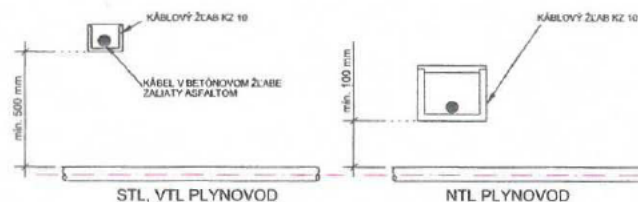
KRIŽENIE TELEKOM. KÁBLA S PLYNOVODOM /STL, VTL a NTL/
