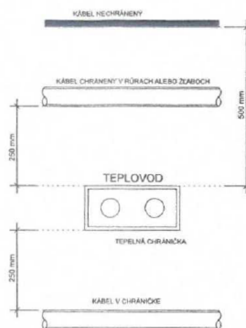
KRIŽENIE TELEKOM. KÁBLA S TEPLOVODNÝM VEDENÍM
