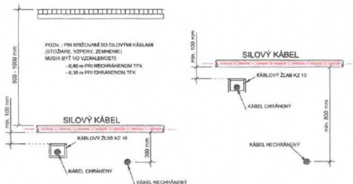
KRIŽENIE TELEKOM. KÁBLA S VODOVODOM A KANALIZÁCIOU
